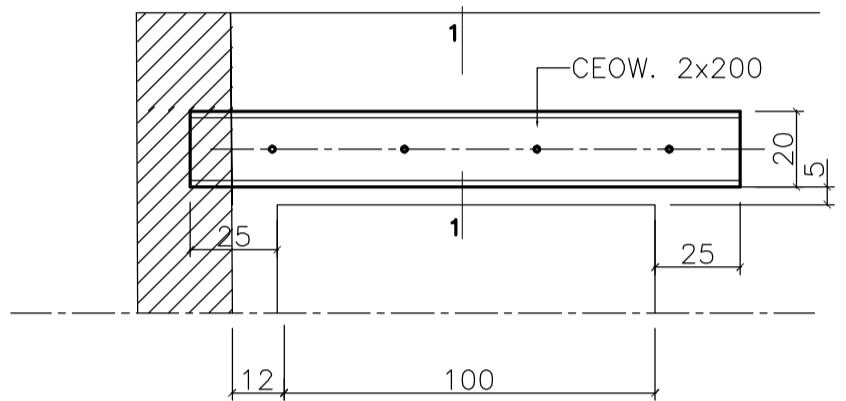
SCHEMAT NADPROŻA DRZWI PROJEKTOWANYCH 1:20
