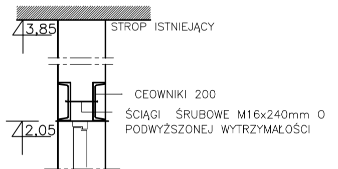
PRZEKRÓJ 1-1 1:20
